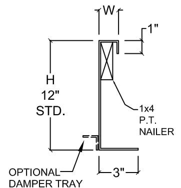
SECTION "A-A" UCC-5
