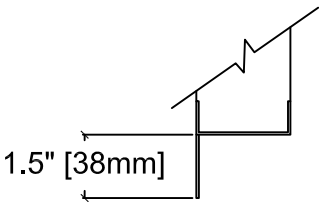
Optional Flange
