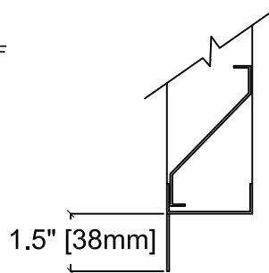
Optional Flange
